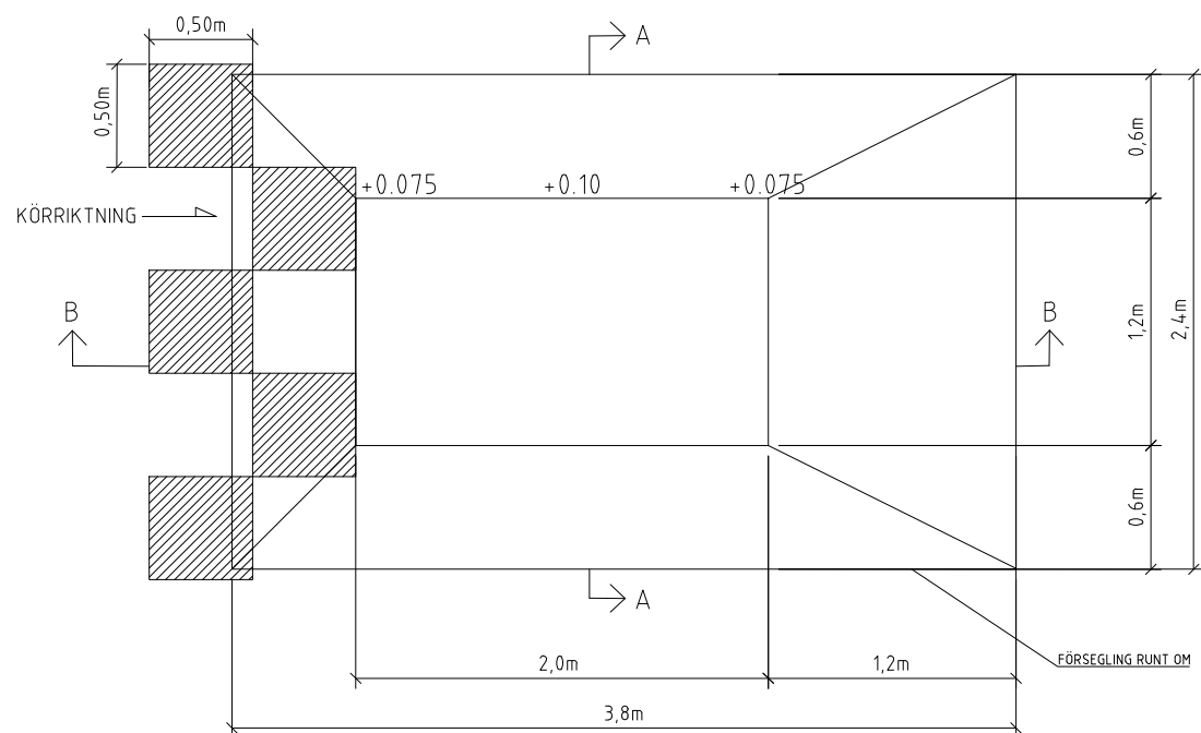
PLAN 1:40
