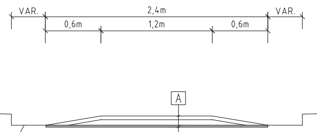
SEKTION A-A 1:40
