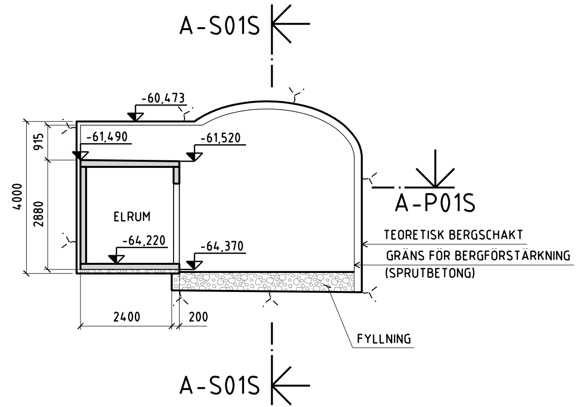
B-S03S SEKTION, ELRUM
