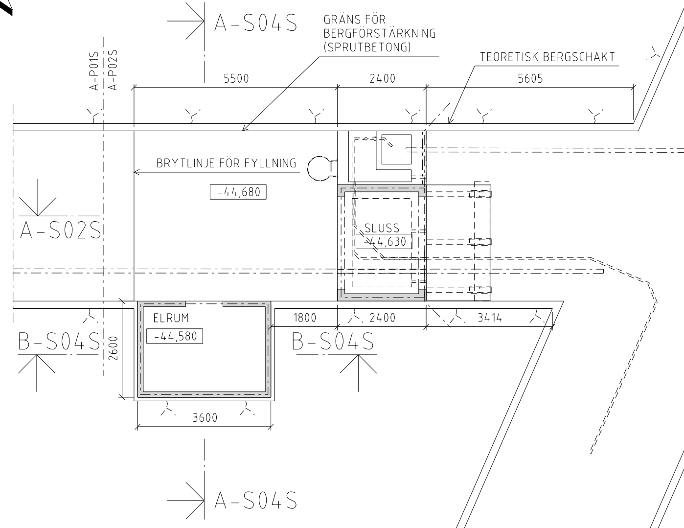
A-P02S PLAN, DJUPANLÄGGNING
