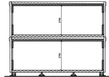
TYPSEKTION M27
